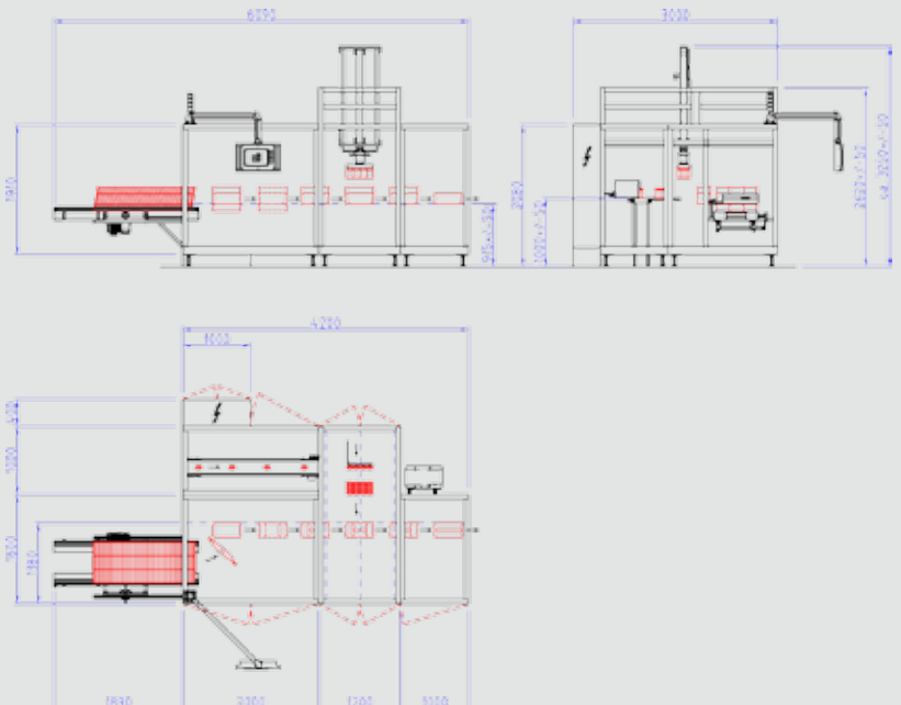
Plan d'ensemble oli 210 V
